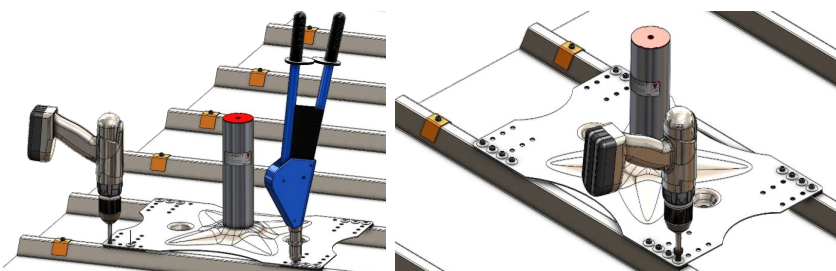
Fixation avec 12 rivets ou 16 vis autoforeuses
